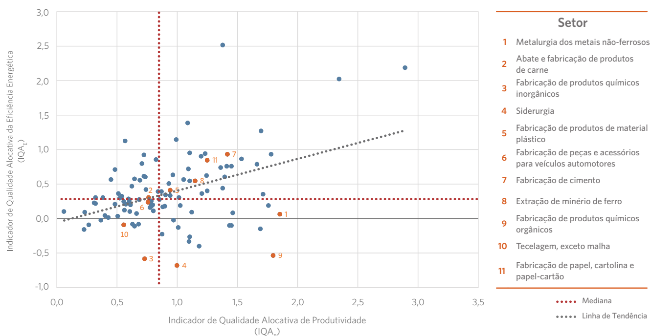
Figura 7: Relação entre o Indicador de Qualidade Alocativa da Eficiência Energética ( IQA_E ) e o da Produtiva ( IQA_P ) em 2015
