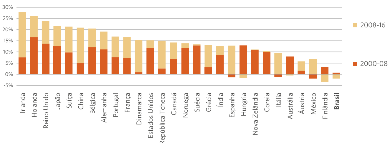
Figura 1: Efeito da eficiência energética em determinados países
