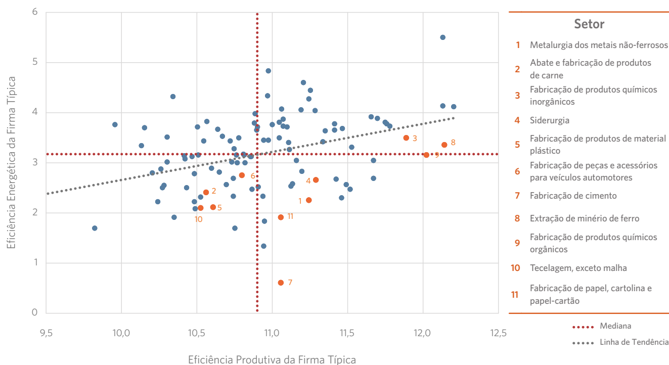
Figura 6: Relação entre as eficiências energéticas e produtivas da firma típica em 2015
